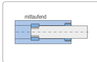
Gleit-Nutenstein, mitlaufend
